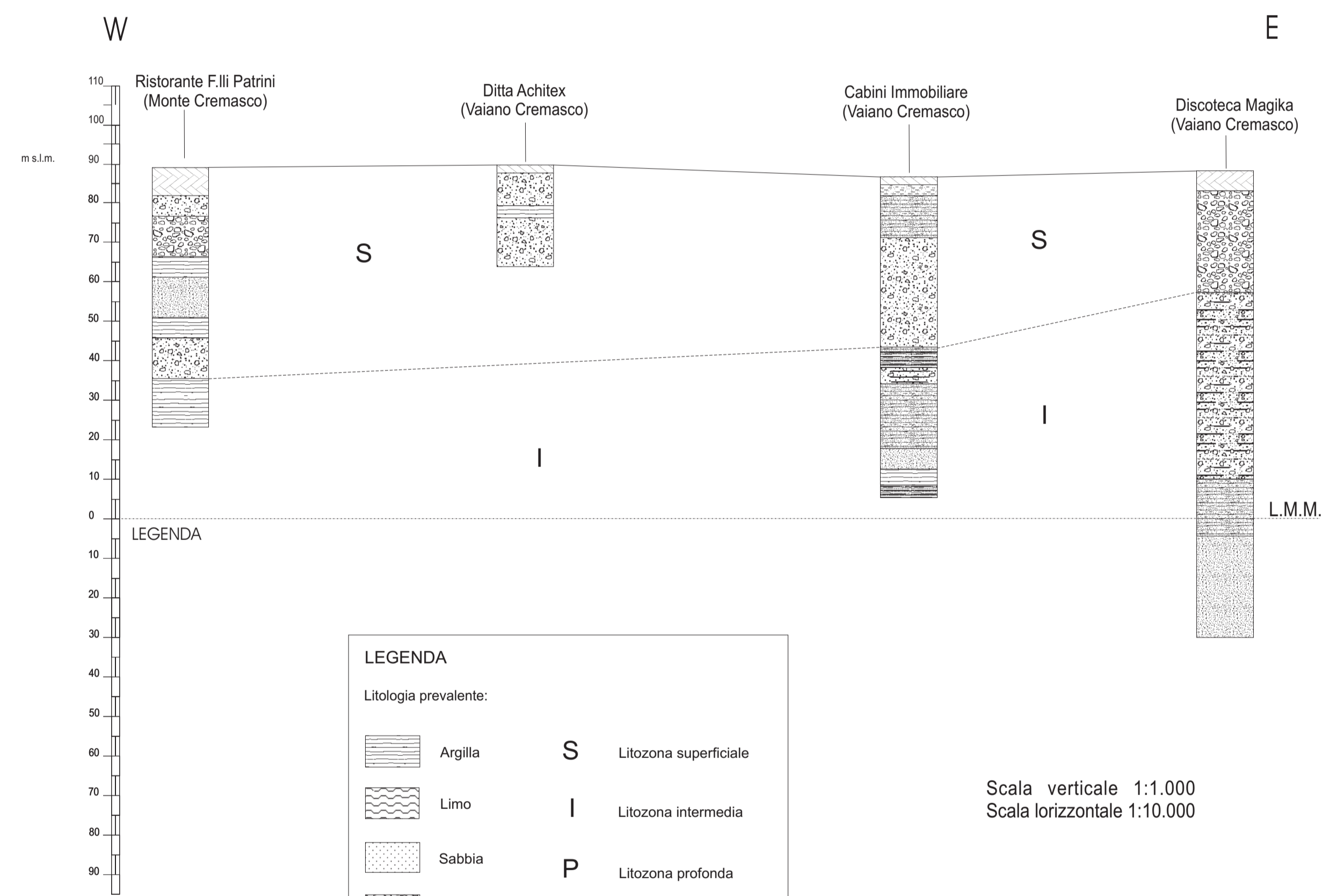
All. 5b SEZIONE GEOLOGICA W - E
