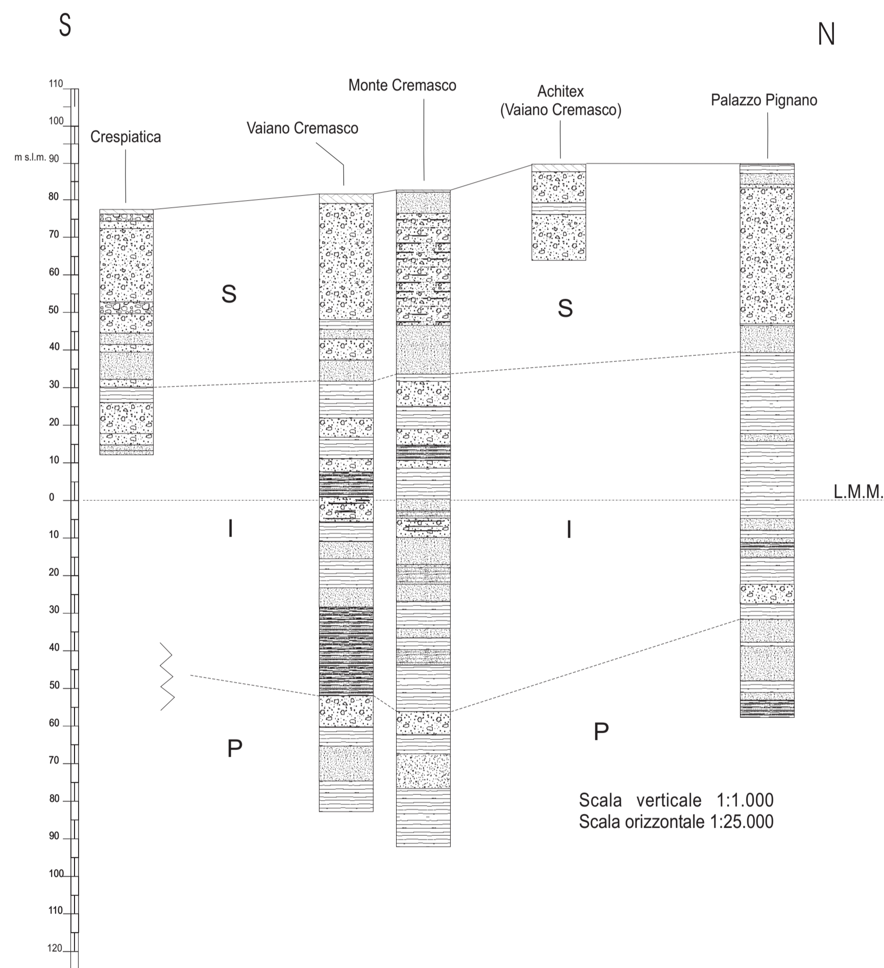
All. 5a SEZIONE GEOLOGICA S - N
